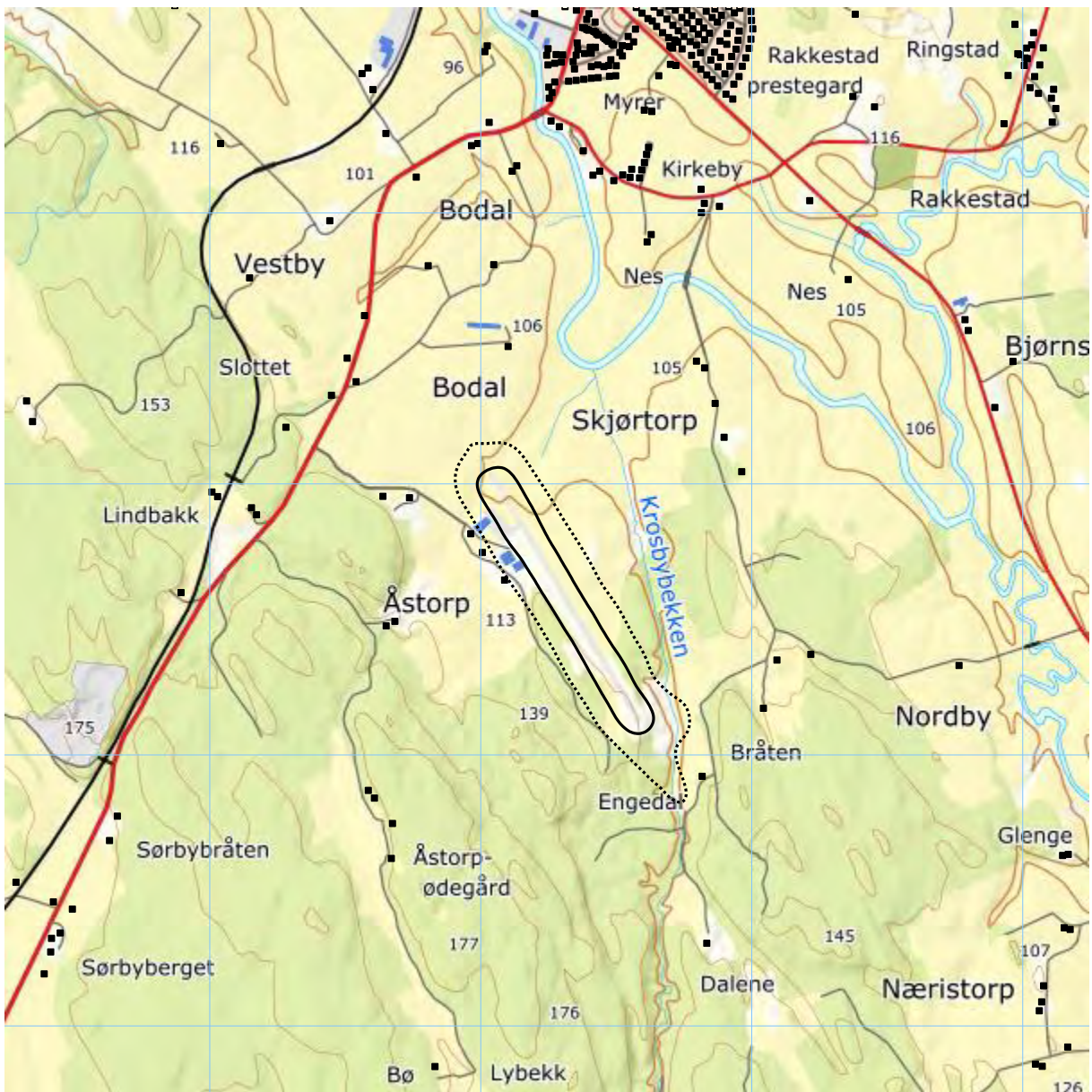
Figur 9-1. Kartleggingsgrense ( L_{Aeq,24h} 57 dB, stiplet strek) og tiltaksgrense ( L_{Aeq,24h} 64 dB, hel strek). M 1:25 000.
