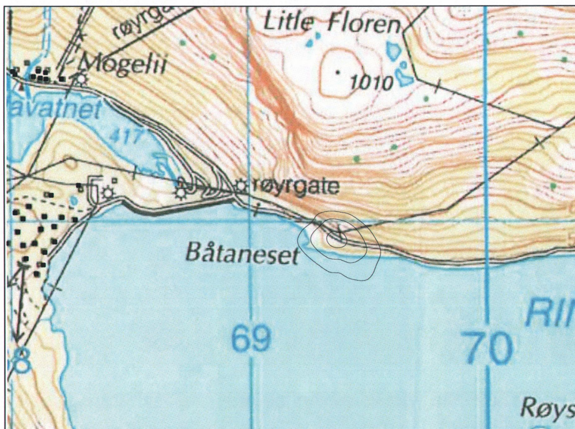
Figur 11-1. Kartleggingsgrenser i henhold til forurensningsforskriften. Koteviser L_{Aeq,24h} 50, 53 og 60 dBA. Målestokk 1:15 000.
